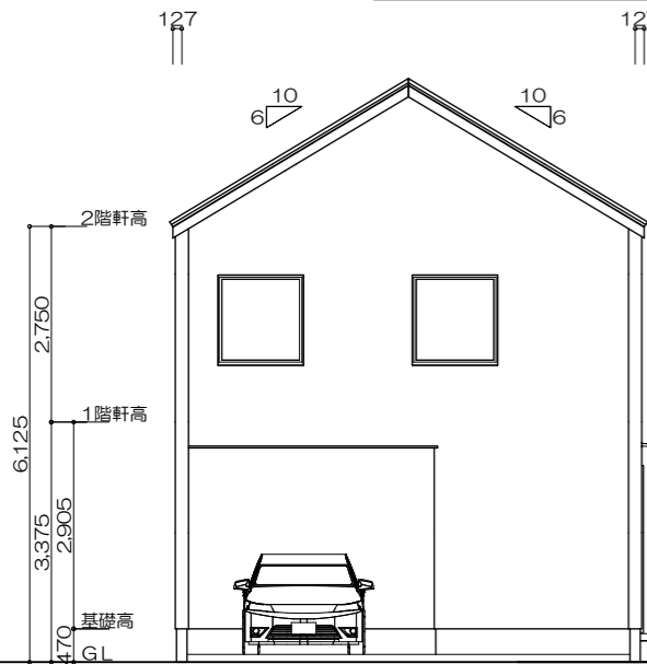
南側 立面図 S:1/100
