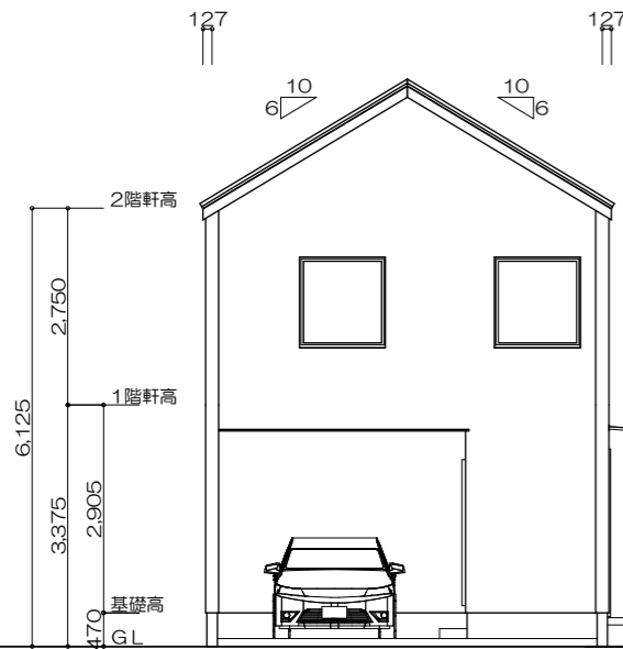
南側 立面図 S:1/100
