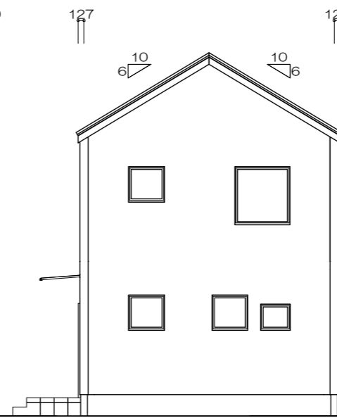
北側 立面図 S:1/100
