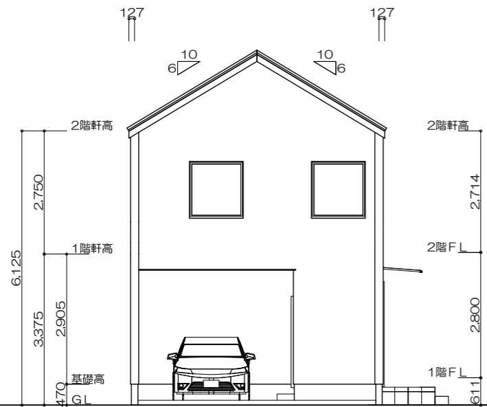
南側 立面図 S:1/100
