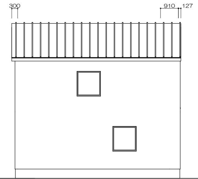
西側 立面図 S:1/100
