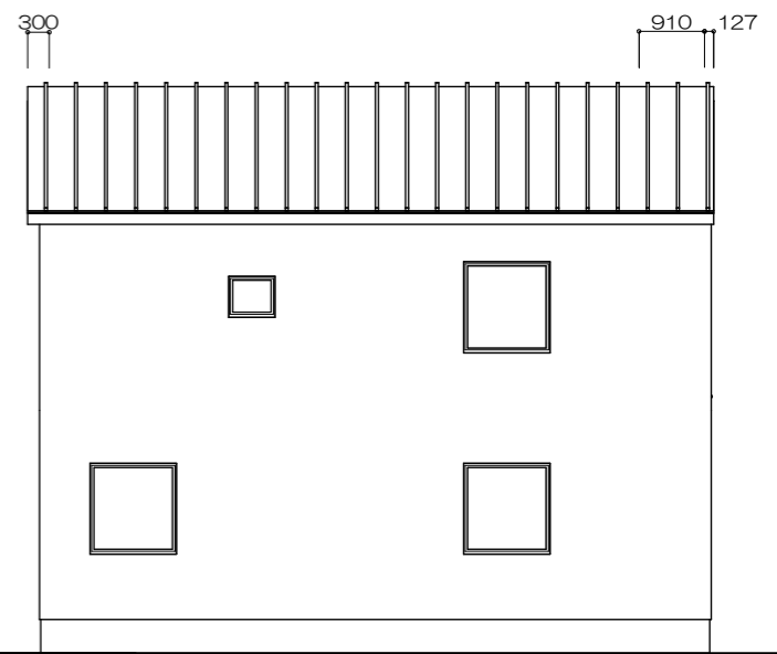
西側 立面図 S:1/100
