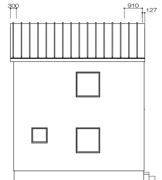
西側 立面図 S:1/100
